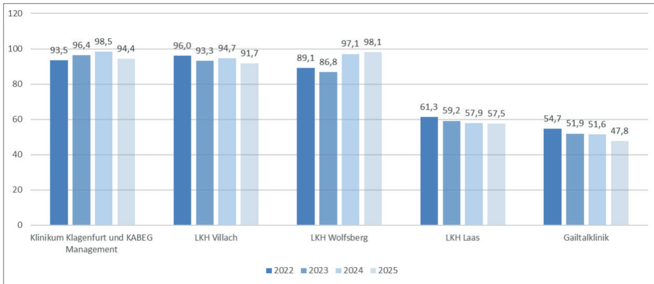
Abbildung 4: Entwicklung des zugekauften Strombedarfs der KABEG-Standorte in kWh pro m 2 Bruttogeschoßfläche 2022-2025
