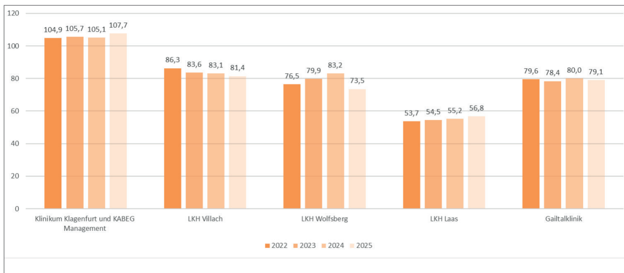
Abbildung 5: Entwicklung des Wärmeenergiebedarfs der KABEG-Standorte in kWh pro m 2 Bruttogeschoßfläche 2022-2025
